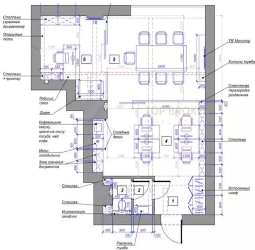
Экспликация помещений
